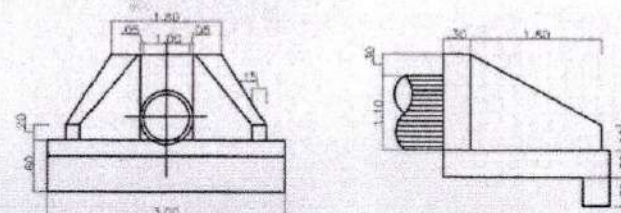
VISTA
