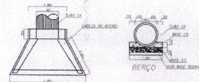
PLANTA BAIXA
