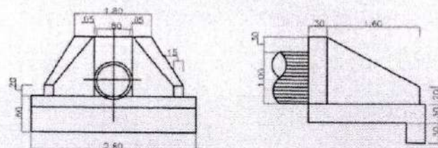
VISTA
